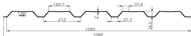
TR 35 plus B - stenový
