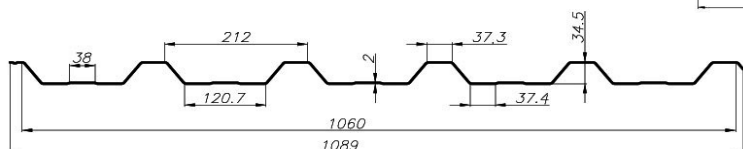
TR 35 plus A - strešný
