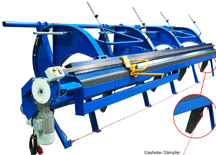
Gasfeder Dämpfer
