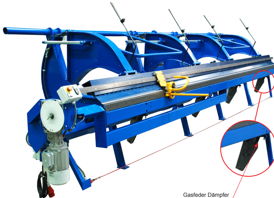
Gasfeder Dämpfer
