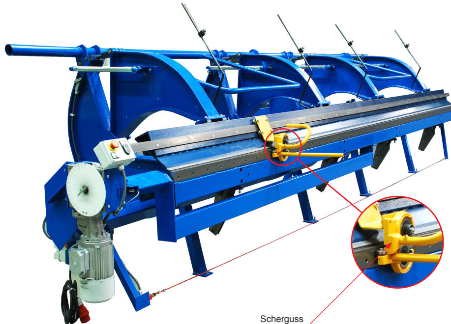
Scherguss
