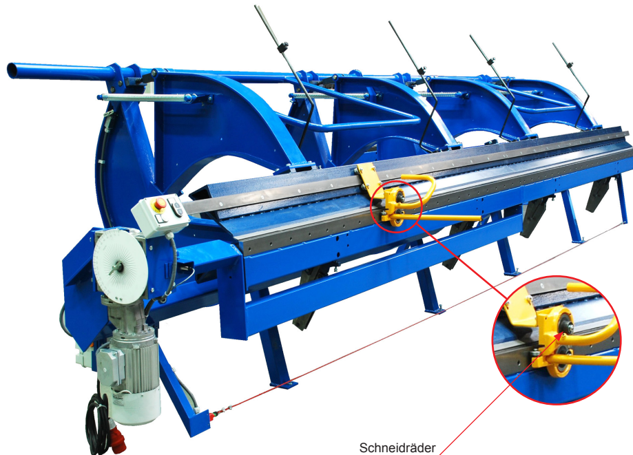
Schneidräder
