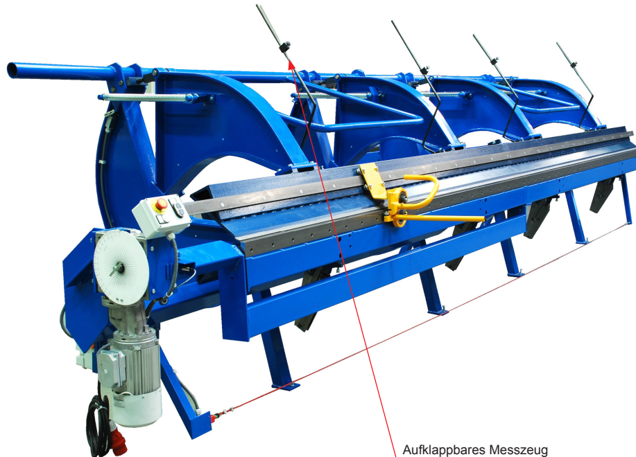
Aufklappbares Messzeug
