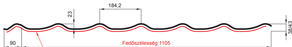
L – MODUL BURKOLAT OPTIM LIS HOSSZ 350 mm
