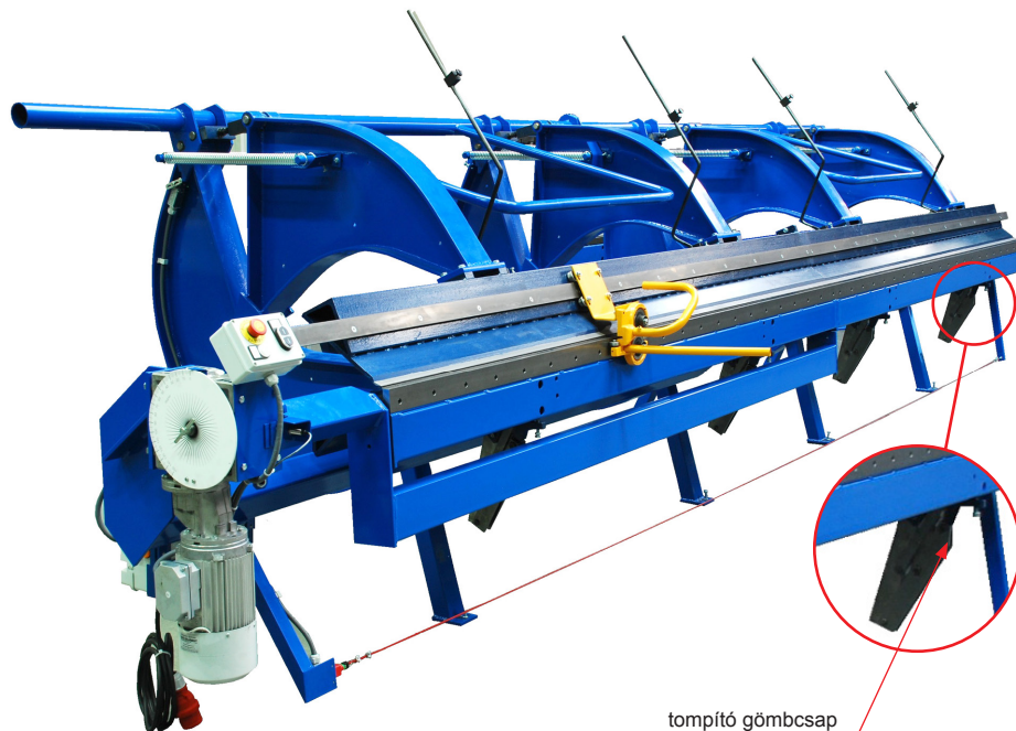
tompító gömbcsap
