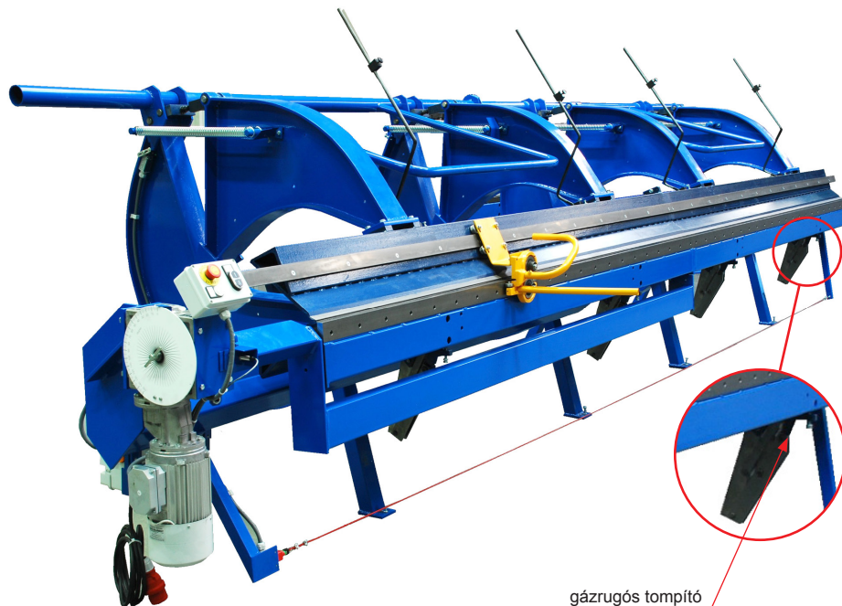
gázrugós tompító
