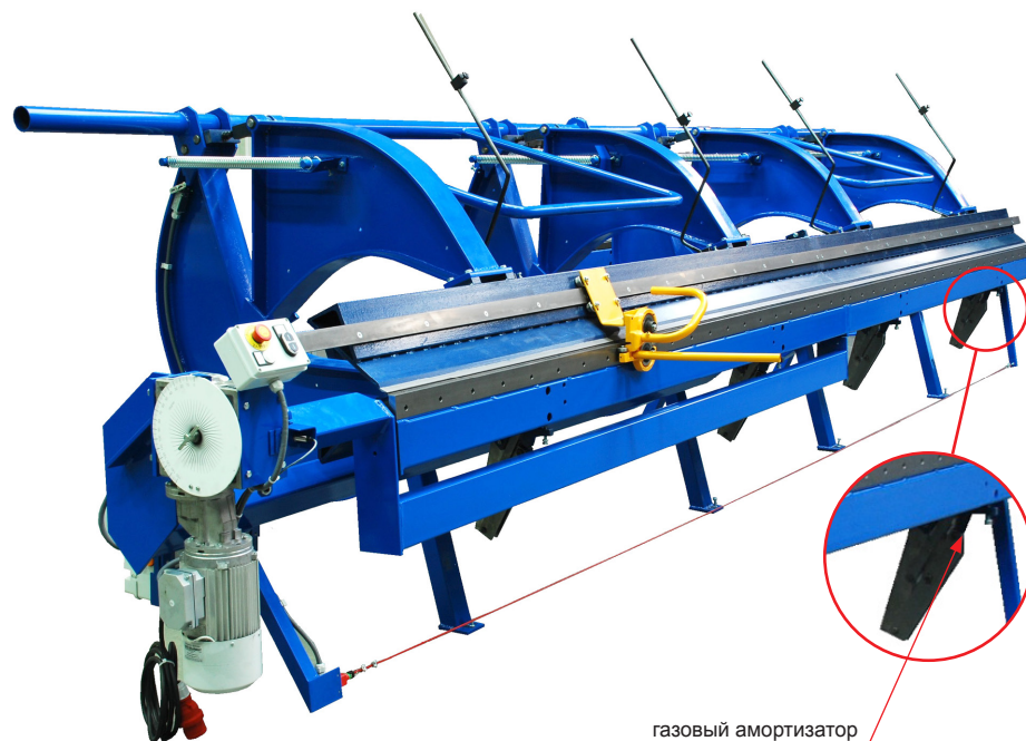
газовый амортизатор
