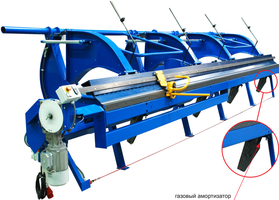
газовый амортизатор
