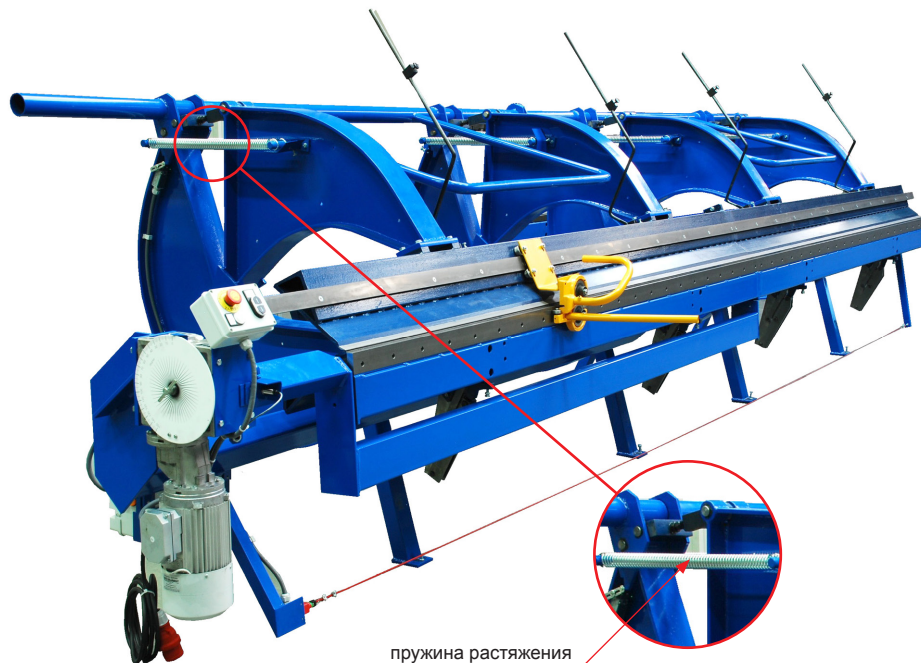
пружина растяжения
