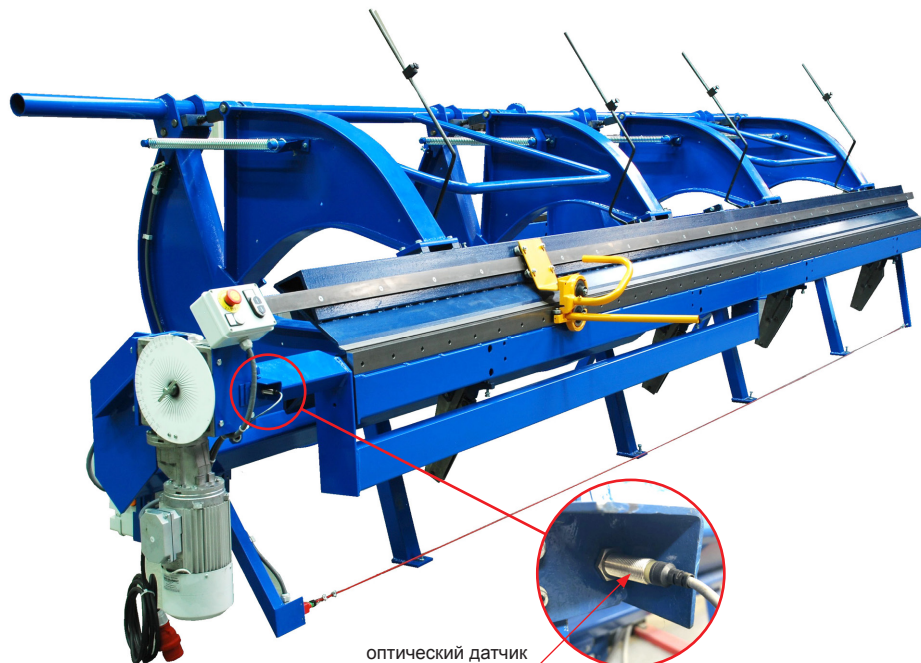
оптический датчик
