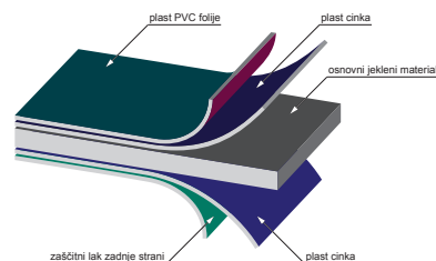
Struktura pločevine:
