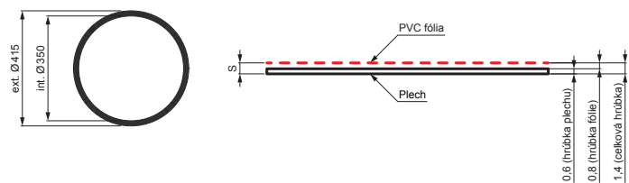
Štruktúra plechu:
