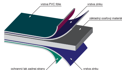
Štruktúra plechu:
