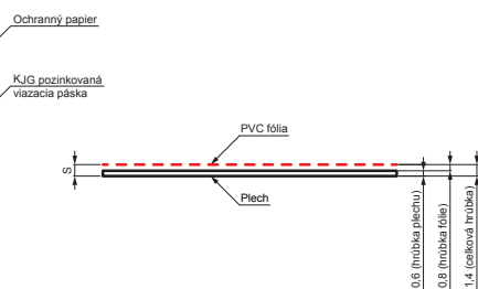
Štruktúra plechu:
