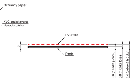
Štruktúra plechu:
