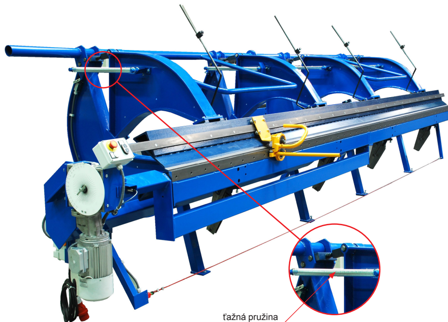
ťažná pružina
