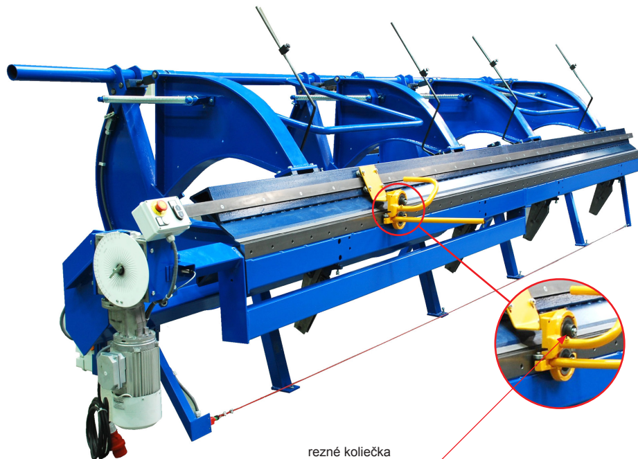
rezné koliečka
