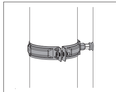
Bilincsfej menetes M10. Beépítés egy teljes téglapéldáján (hőtechnikai követelmények nélkül).
