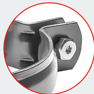
ROHRSCHELLE M10 EDELSTAHLSCRAUBE M8x30 (Aluminium, Edelstahl)
