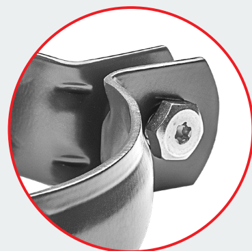
OBJEMKA M10 INOX VIJAK M8x30 (Aluminij, Inox)
