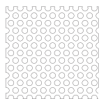
Voľný prierez Ao 46% Ø otvoru 5 mm
