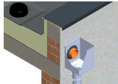
2. Spôsob montáže kotlíka zberného excentrického
