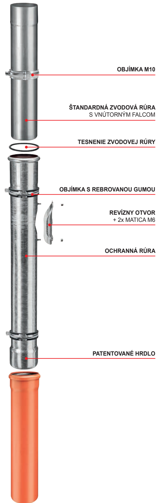
VERZIA B PVC KANALIZAČNÁ RÚRA
