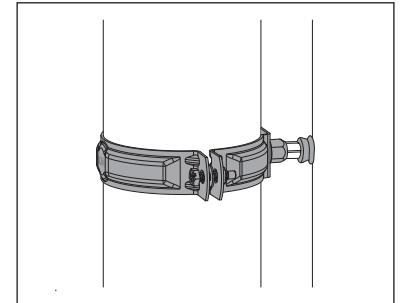
Zvodová objímka M10. Montáž na príklade plnej tehly (bez termických požiadaviek)
