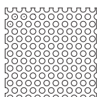
Volný prierez Ao 46% Ø otvoru 5 mm
