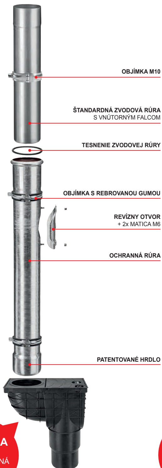
VERZIA B PVC KANALIZAČNÁ RÚRA
