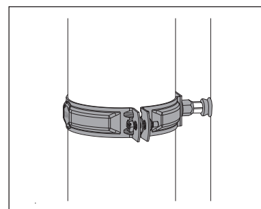
Zvodová objímka M10. Montáž na príklade plnej tehly (bez termických požiadaviek)
