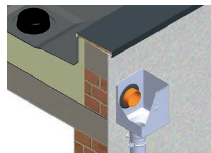
2. Spôsob montáže kotlíka zberného exzcentrického
